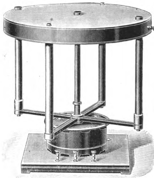
FIG. 192.—RECTIFIER FOR RÖNTGEN-RAY WORK (Schall).
