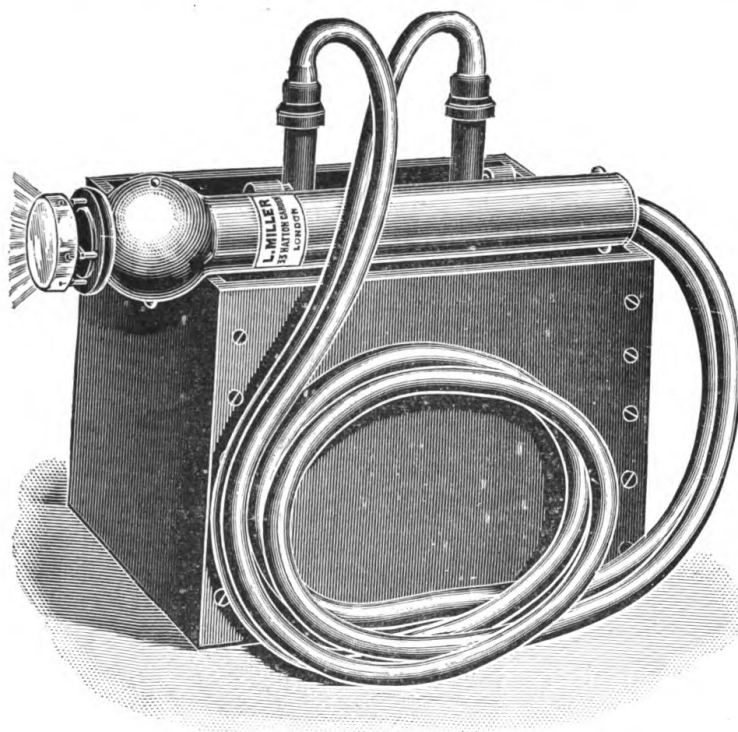
FIG. 188.—CONDENSER SPARK LAMP.
