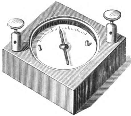
FIG. 39.—GALVANOSCOPE.
