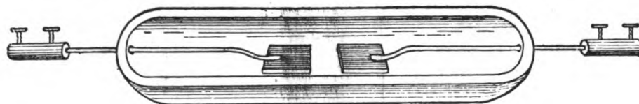
FIG. 55.—SIMPLE LIQUID RHEOSTAT.
