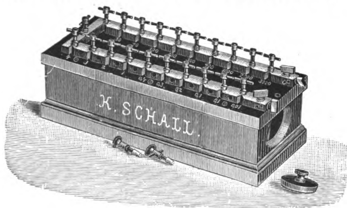
FIG. 53.—PLUG RHEOSTAT.
