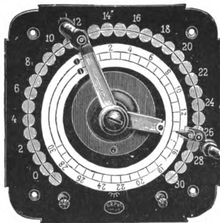
FIG. 48.—DOUBLE COLLECTOR.
