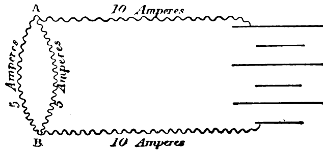
FIG. 40.—DIVIDED CIRCUIT.
