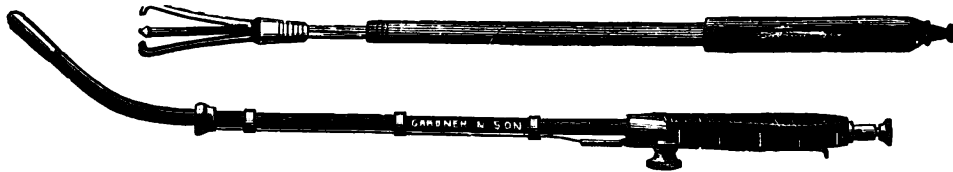
FIG. 124.—DR. MILNE MURRAY'S ELECTRODE.
