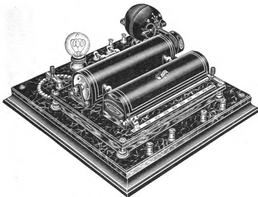
Fig. 12.—Multiplex. (Victor.)
