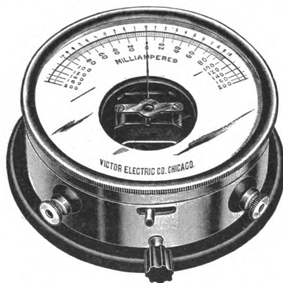
Fig. 10.—Milliampèremeter. (Victor.)
