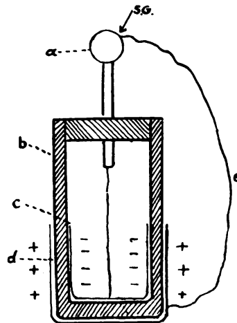
Fig. 40.—A Leyden jar.
